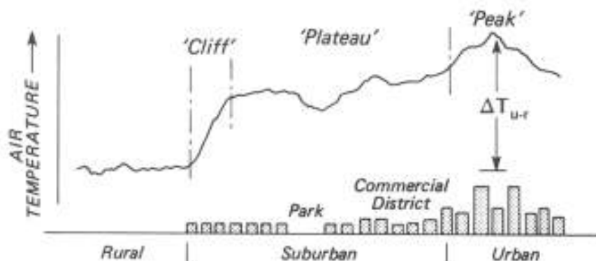
Τυπική σχηματική απεικόνιση της αστικής θερμικής νησίδας (Oke, 1987)
